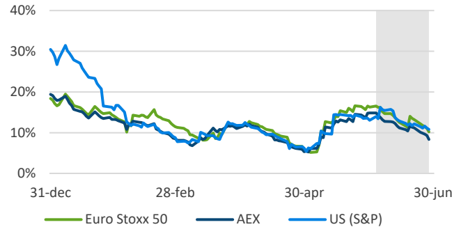
Geïmpliceerde volatiliteit
